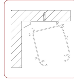
Tavan Montajı
