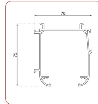
Zmkp Üst Profil Kesit
