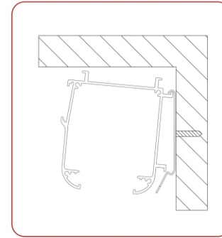
Duvar Montajı
